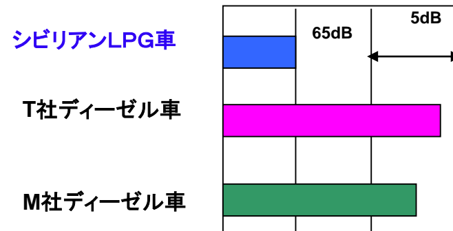
3,000rpm一定速時騒音
